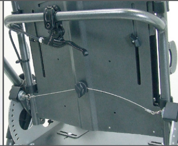
basculement aisé de l'assise et du dossier
