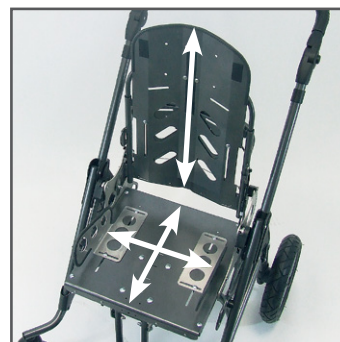
hauteur dossier, largeur et profondeur d'assise
